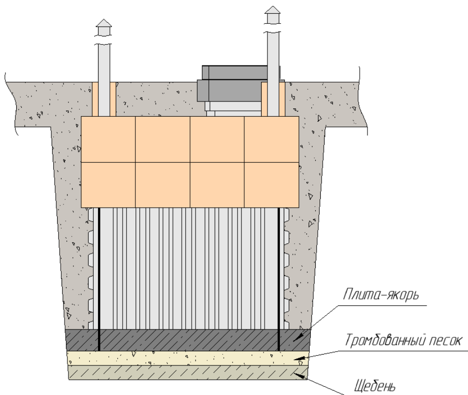
Схема монтажа погребов Т1500 с нижним якорением
