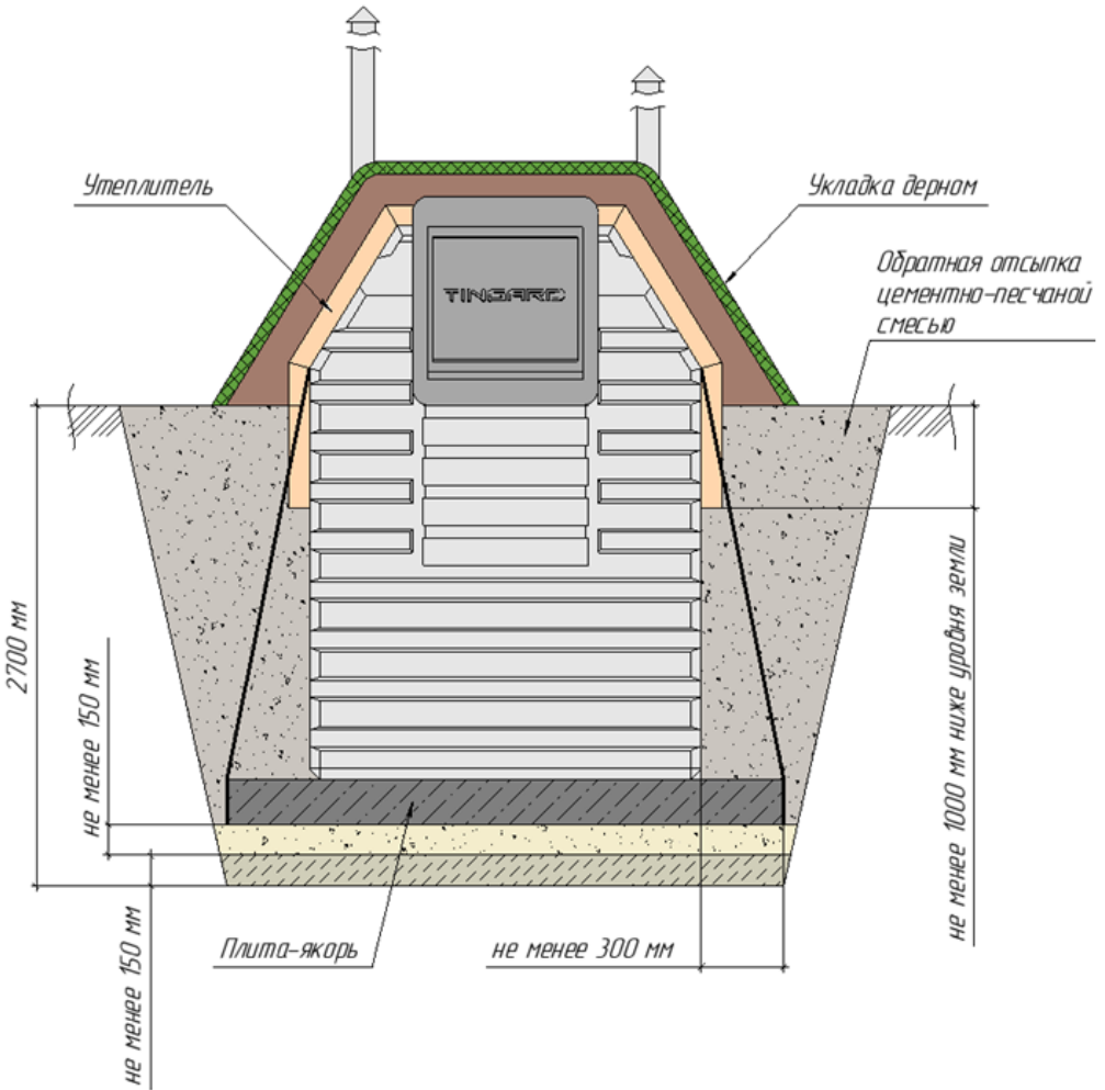
Схема монтажа погреба Т1900Б, Т2500Б
