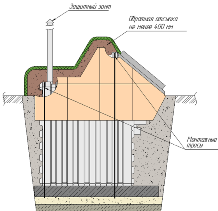
Схема монтажа погребов Т1900Б, Т2500Б
