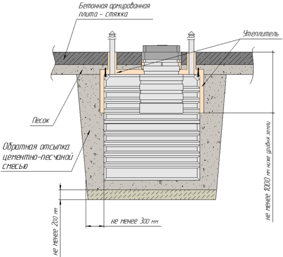
Схема монтажа погреба Т1900К, Т2500К с верхним якорением
