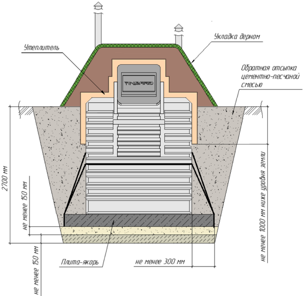
Схема монтажа погребов Т1900БК, Т2500БК
